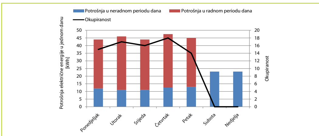
Slika 6-1: Primjer prikaza dnevne potrošnje električne energije po funkcijskim periodima i razine okupiranosti u odabranom sedmici
