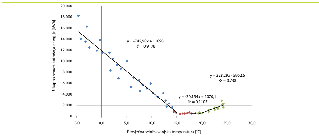
Slika P-14: Primjer E-T krivulje ukupne energije sa silaznim zimskim razdobljem, prijelaznim razdobljem i uzlaznim ljetnim razdobljem
