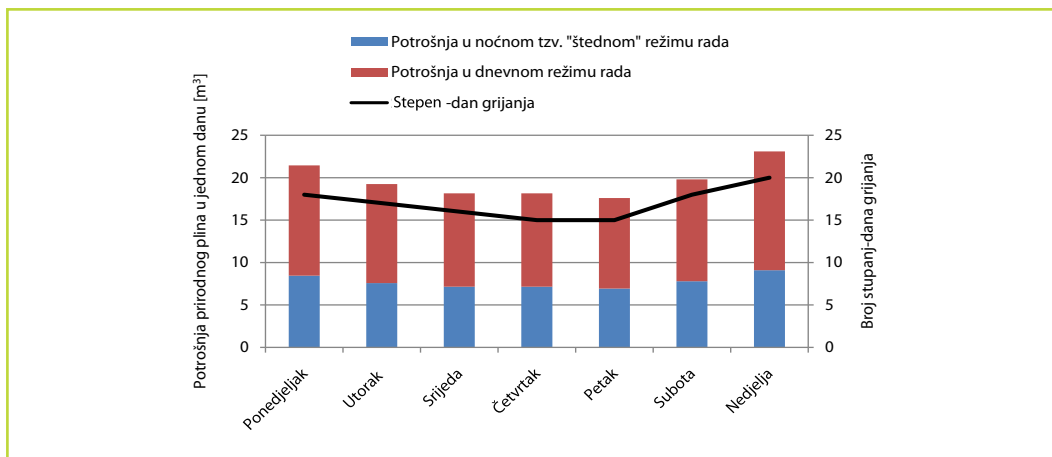
Slika 6-2: Primjer prikaza dnevne potrošnje prirodnog gasa po funkcijskim periodima i stepen-dana grijanja u odabranom sedmici
