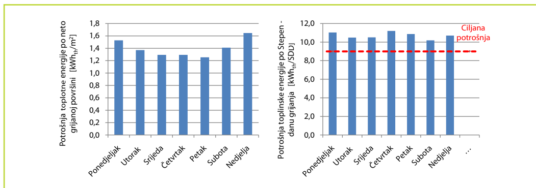
Slika 6-5: Primjer prikaza dnevne potrošnje toplote energije po neto grijanoj površini (lijevo) te po stepen-danu grijanja s određenom ciljanom nivoom potrošnje (desno)
