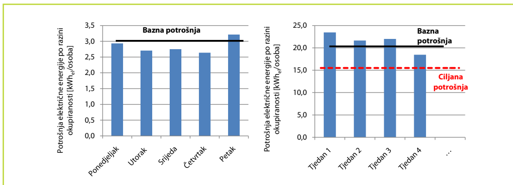
Slika 6-4: Primjer prikaza potrošnje električne energije po nivou okupiranosti po danima u sedmici (lijevo) te po tjednima s određenom ciljanom nivoom potrošnje (desno)
