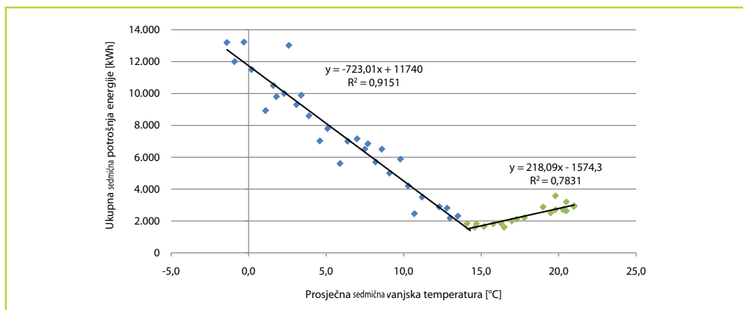
Slika P-12: Primjer E-T krivulje ukupne energije sa silaznim zimskim razdobljem i uzlaznim ljetnim razdobljem
